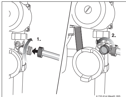
Sl. 4 Priključitev cevi
